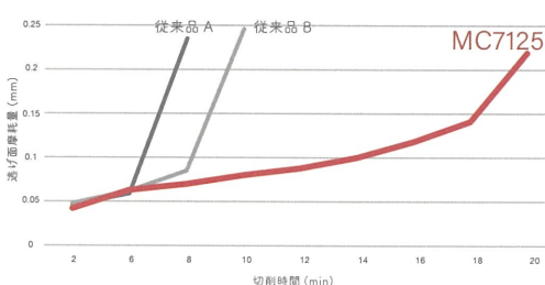
SUS304 断続加工比較
