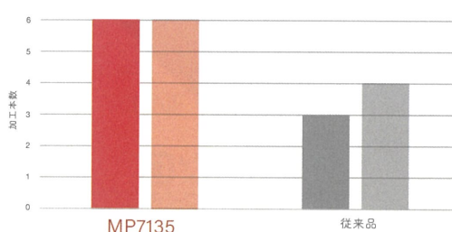
SUS304 断続加工比較
