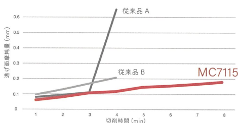
SUS316L 湿式切削加工耐摩耗性試験
